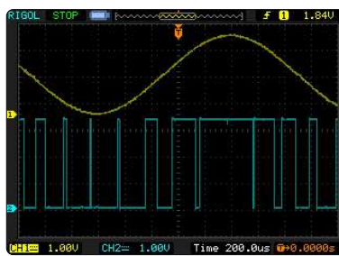
PWM Output
